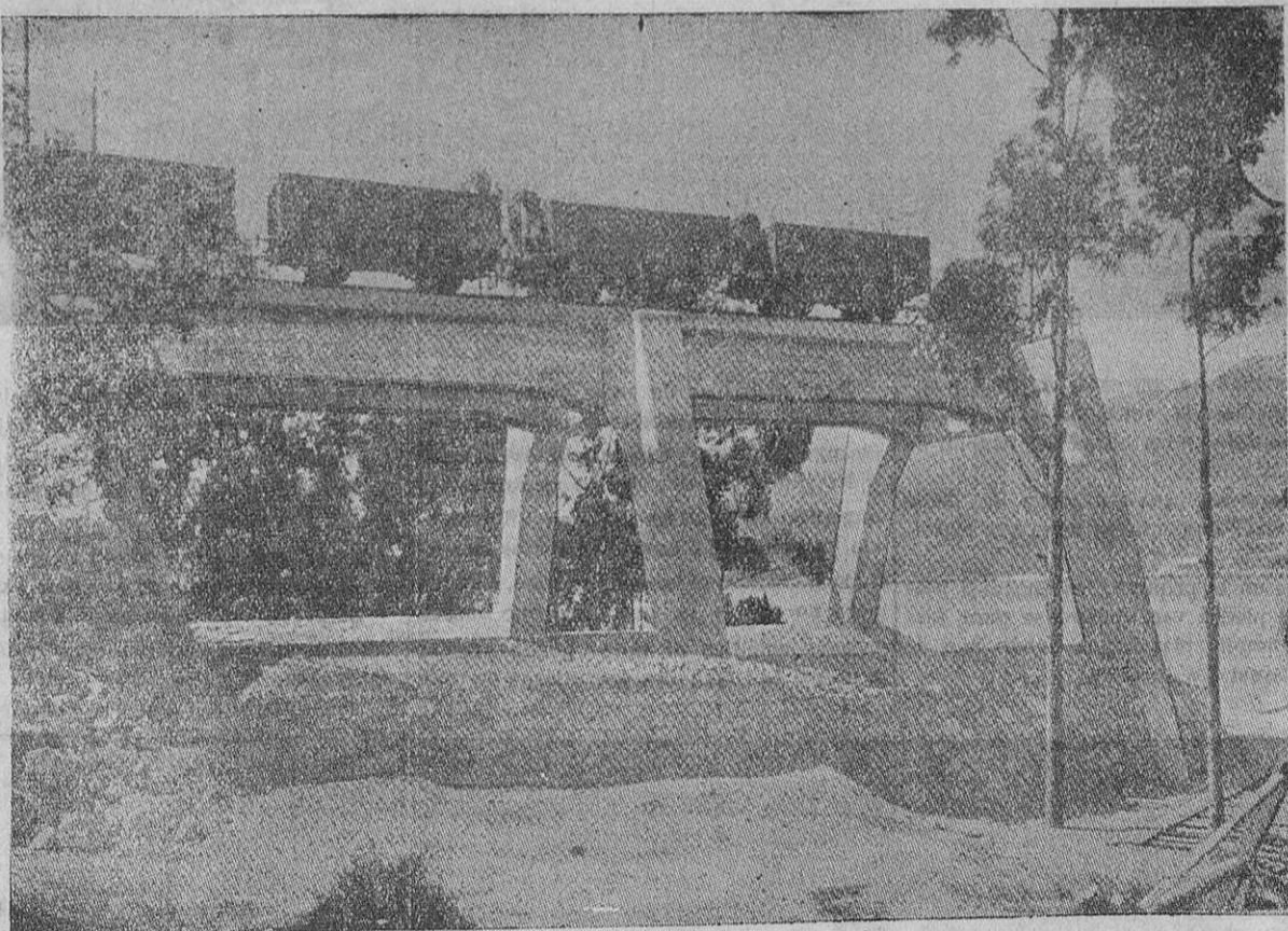
Puente del cargadero de mineral de Rande (Vigo) construido de cemento armado, capaz de resistir más de 20.000 toneladas de peso en el cual se empleó única y exclusivamente el
